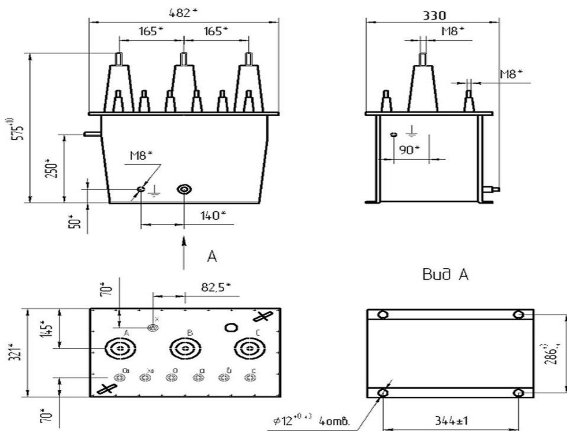
fig.1 Transformator de tensiune solicitat, la tensiunea de 10kV.
