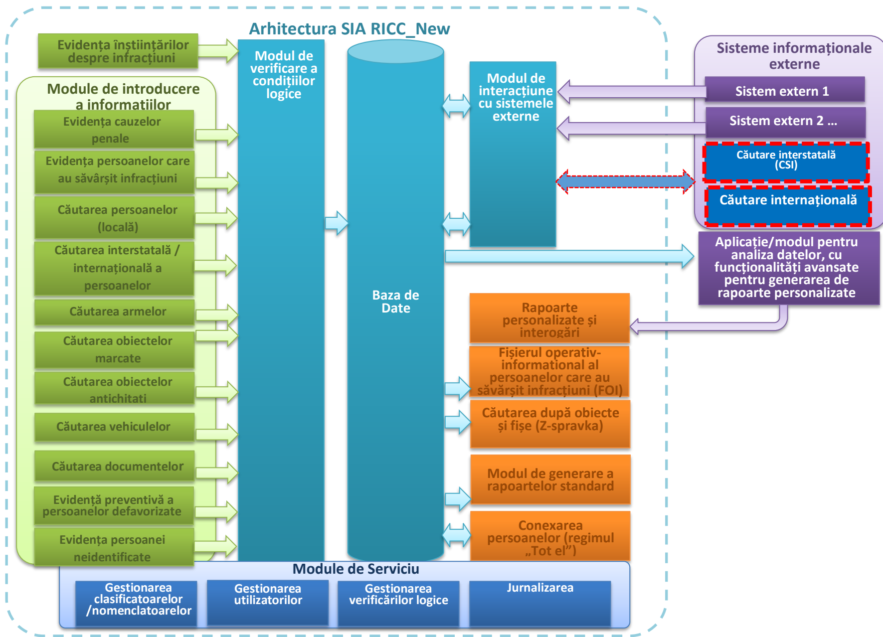
Fig. 4. Diagrama Arhitecturii SIA RICC după procesul de reinginerie
