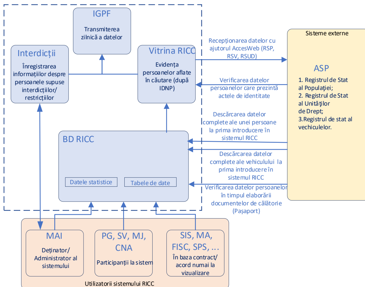
Fig. 1. Interacțiunea actuală a "RICC Old" cu sistemele informaționale
