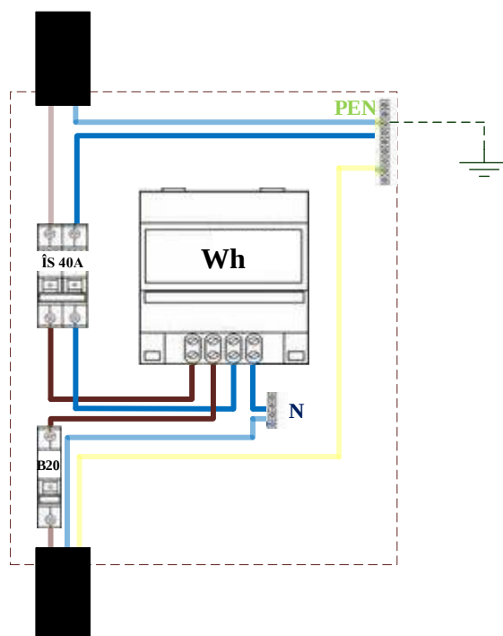
Schema electrică acestuia
