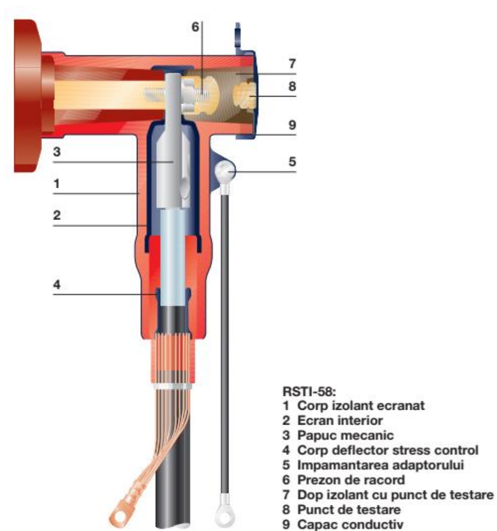
Desenul constructiv al adaptorului terminal în T
