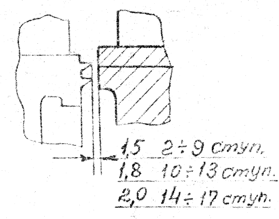
III M 1:1 2+17 ступени
