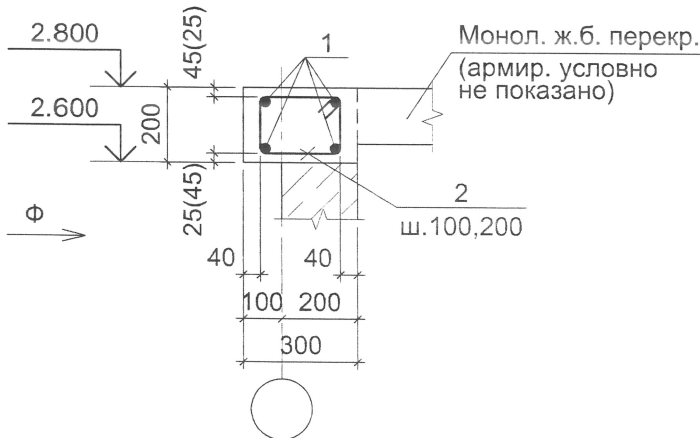
3 - 3
