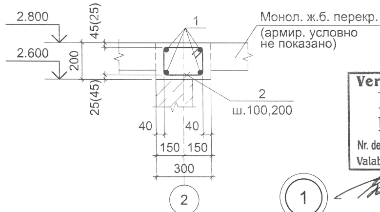
2 - 2 (Пояс ПСм-1)
