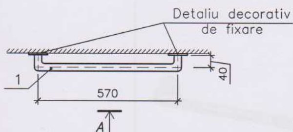
Vedere A
