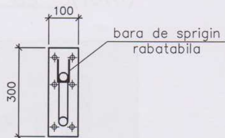
Vedere B
