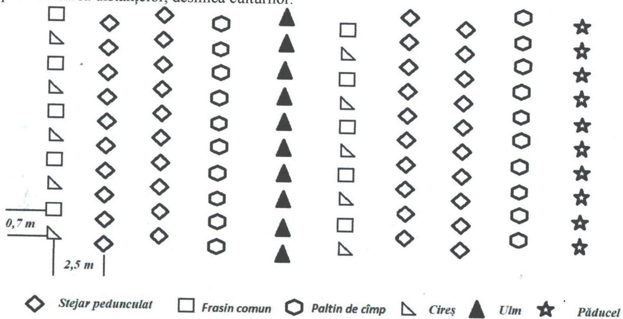
Fig. 3.2. Amestecul în benzi și dispozitivul de plantare în paralelogram
