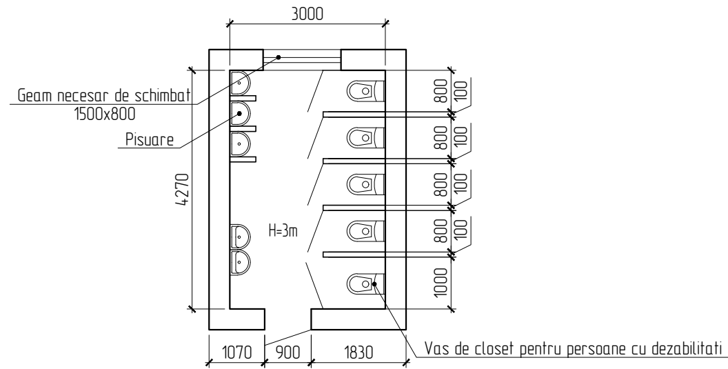
Bloc A Etajul 1 Baieti Sc.1:100
