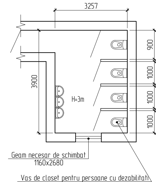
Bloc A Etajul 3 Fete Sc.1:100
