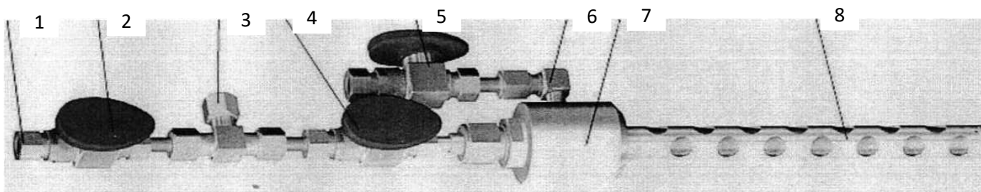
Figura 2 - Conducta liniei de picurare; 2 - Robinet de izolare; 3 - Conducta de injecție, 4 - Robinet de izolare; 5 - Ventil de izolare al panoului pneumatic; 6 - Conducta de prelevare a gazului din panoul pneumatic; 7 - Cuplaj; 8 - Evaporator.
