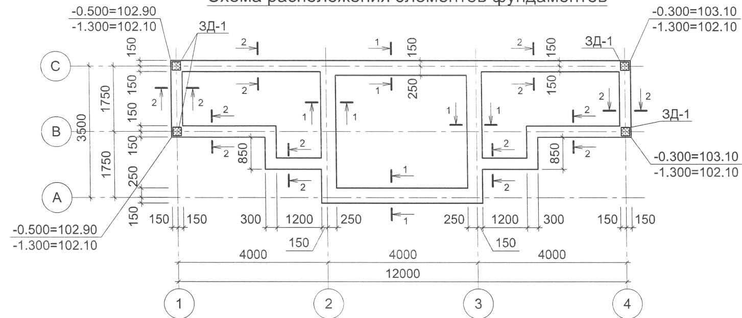
Схема расположения элементов фундаментов
