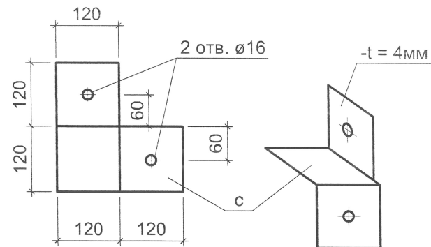
Соединительная деталь МД-1
