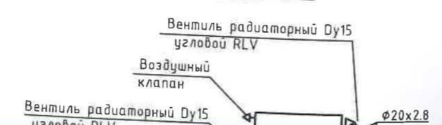
Схема узла "Б"
