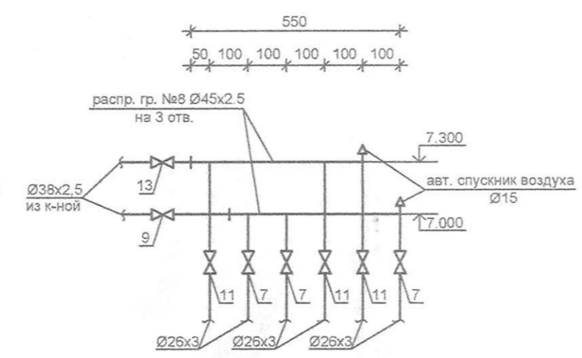
Распределительная гребенка №8
