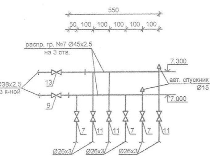
Распределительная гребенка №7
