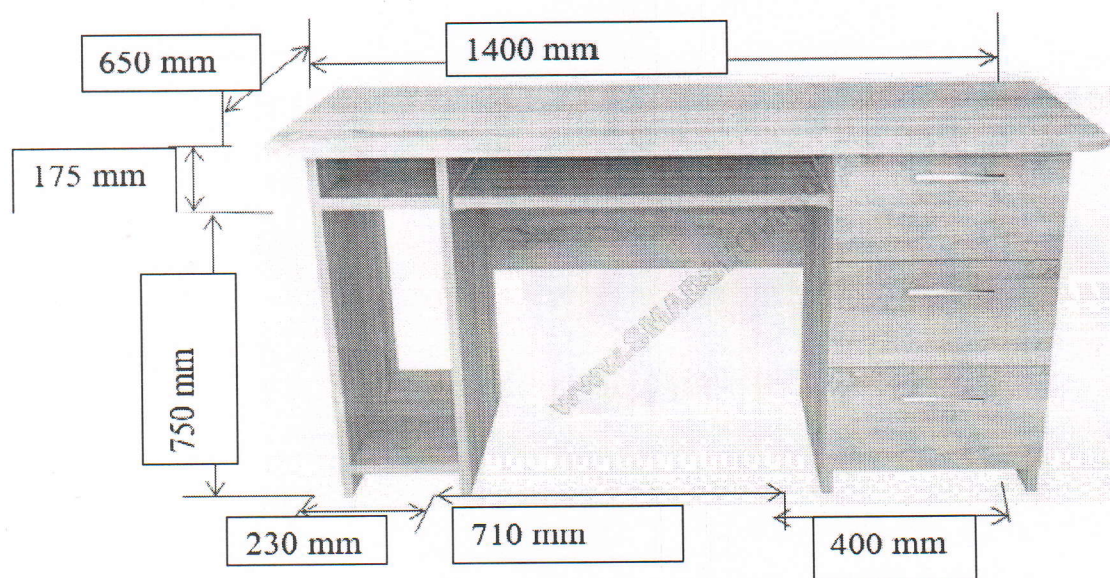
Fig.4 Masă de birou cu sertare încorporate
