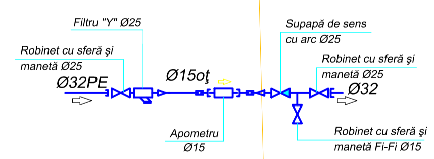
Schema de montare a nodului apometric pentru vizeu cu apometru Ø15 (cam. A-4)
