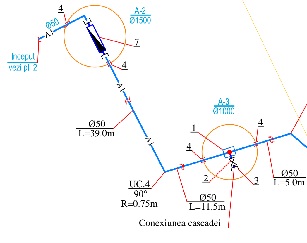
Detalierea rețelei de apeduct în parc
