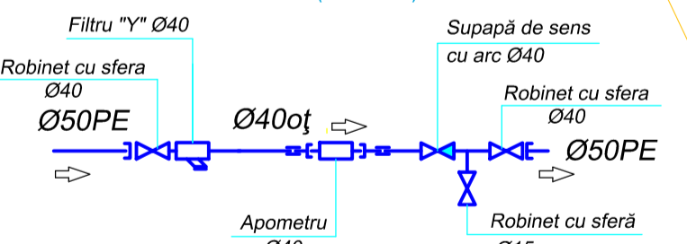
Schema de montare a nodului apometric proiectat cu apometru Ø40 cu transmiterea datelor la distanță (cam. A-2)
