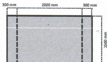
secțiune 1-1
