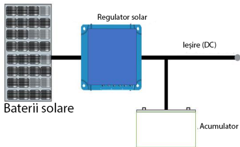
Figura1. Schema centralei autonome de curent continuu.
