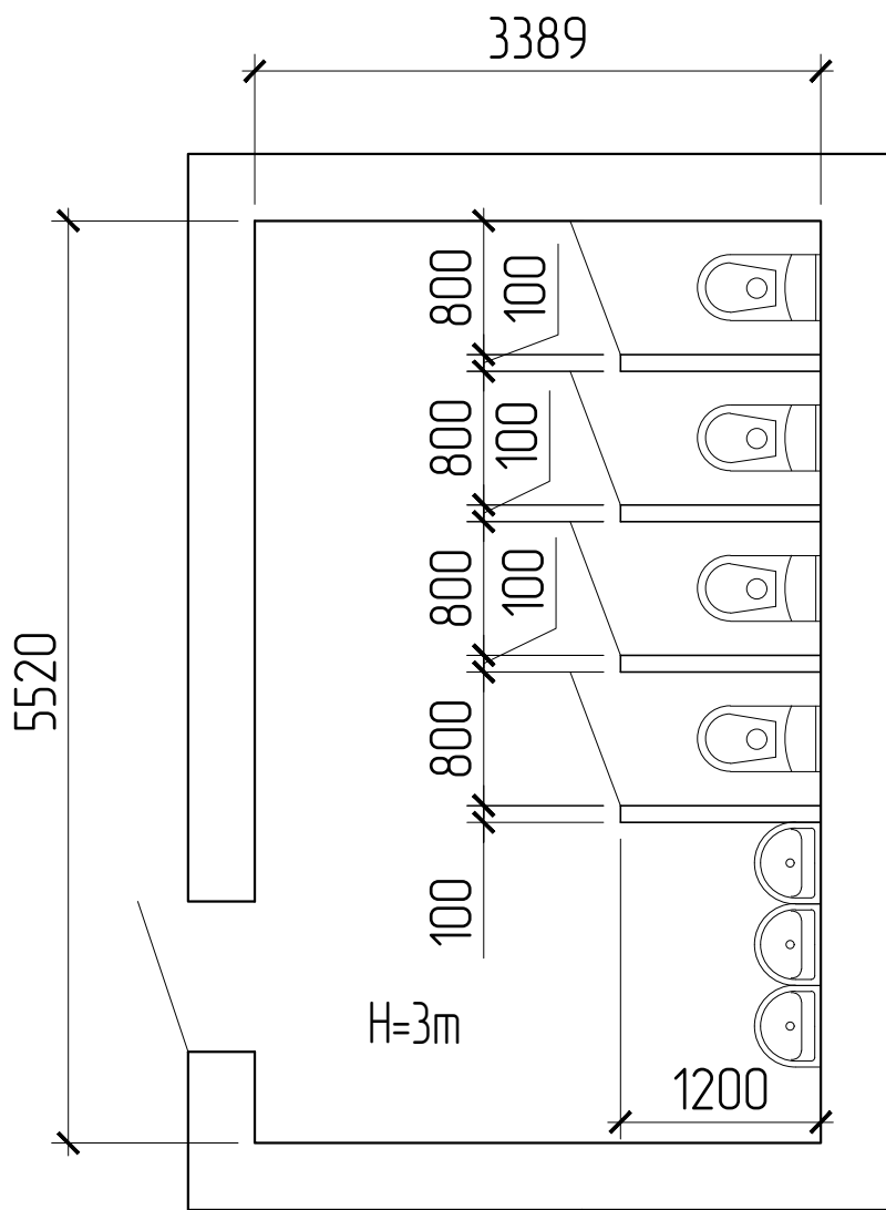
GTS Nr.2 Etajul 2 Sc.1:100
