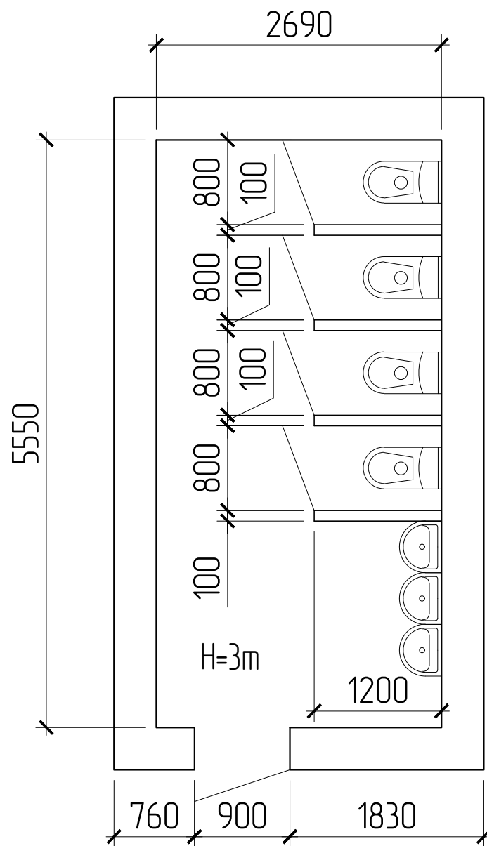
GTS Nr.1 Etajul 2 Sc.1:100
