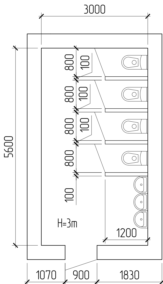
GTS Nr.5 Etajul 2 Sc.1:100
