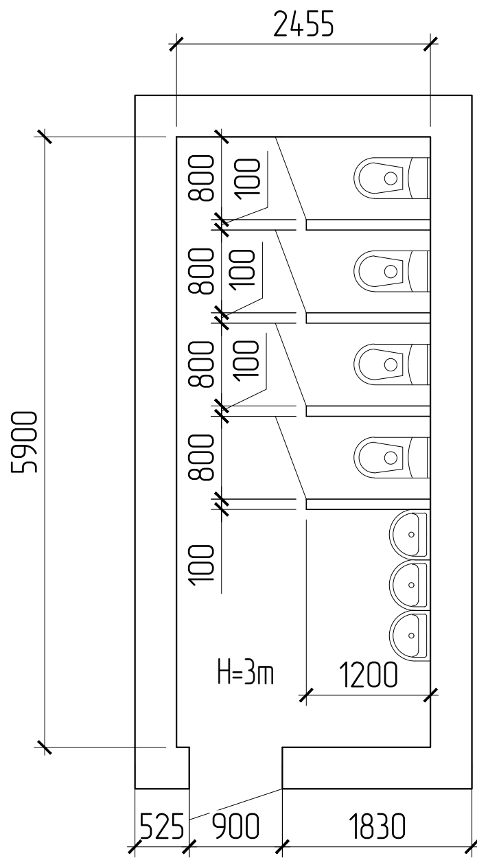
GTS Nr.4 Etajul 2 Sc.1:100
