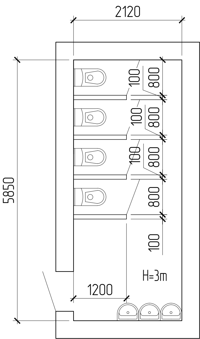
GTS Nr.7 Etajul 2 Sc.1:100
