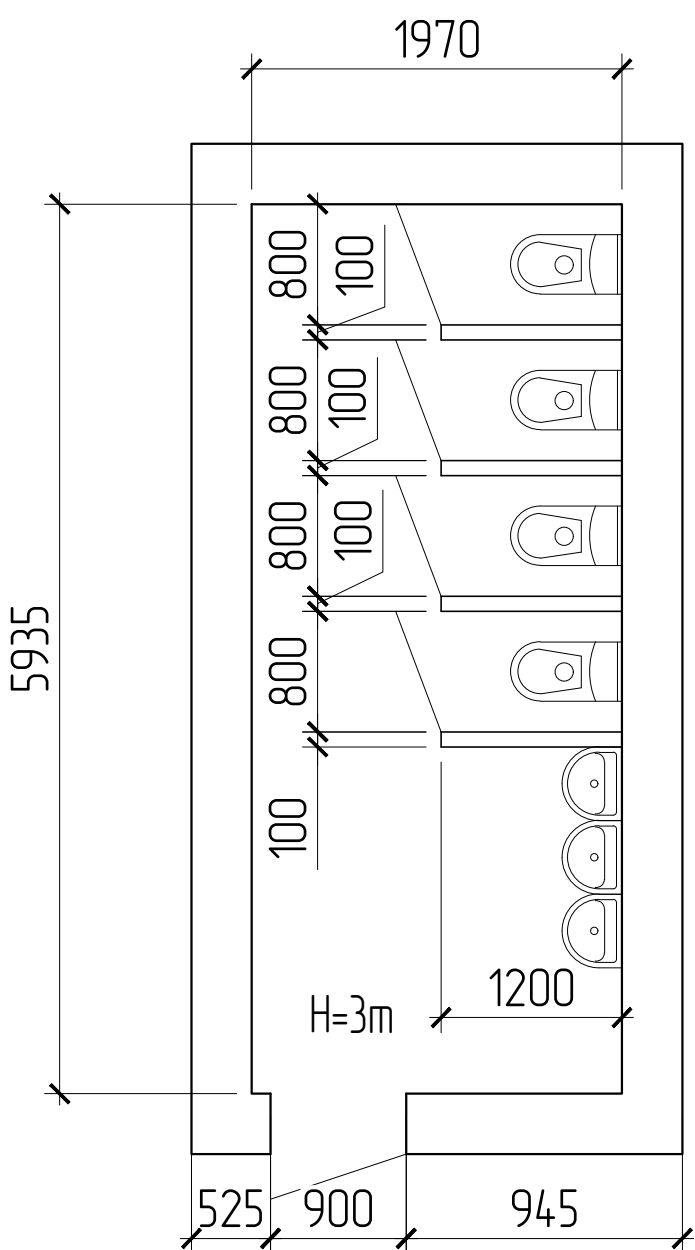
GTS Nr.6 Etajul 1 Sc.1:100
