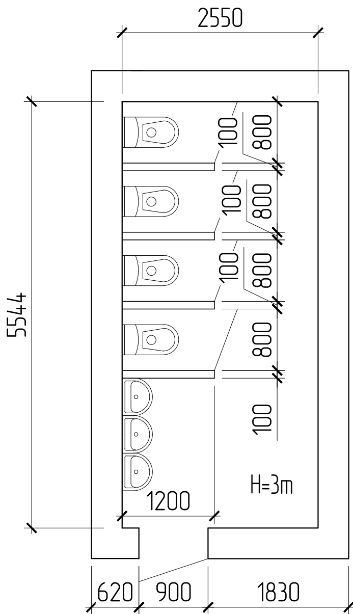
GTS Nr.3 Etajul 1 Sc.1:100
