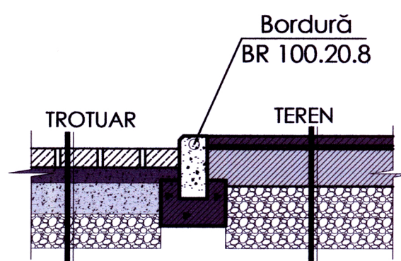
NODUL DE MONTARE A PAVAJULUI TROTUARELOR SI A TERENURILOR DE JOACA SI BASCHET
