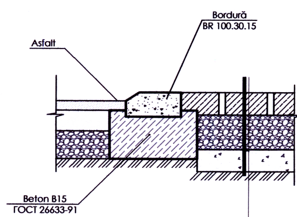
NODUL DE MONTARE A PAVAJULUI PARCARII AUTO SI ASFALT
