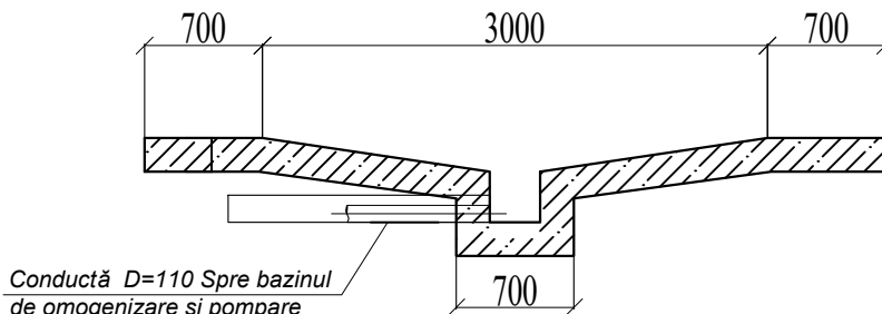
Sectiune 1-1
