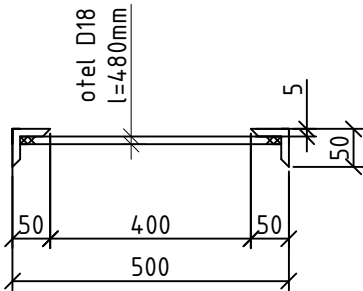
SECTIUNEA 1-1
