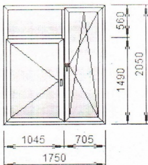
Unitate de fereastră 1750x2050
