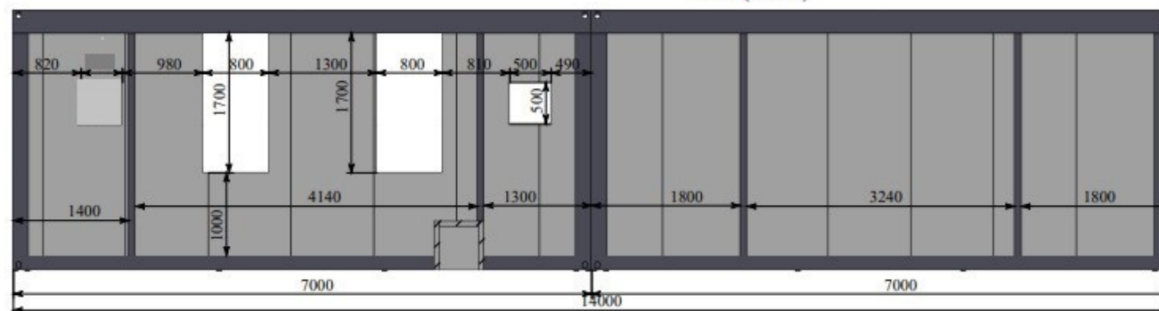
A-A (1 : 55)
