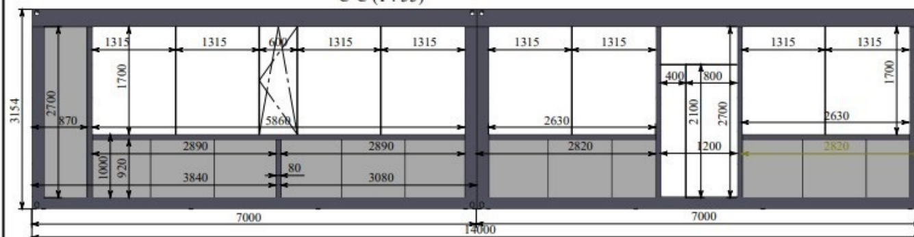
D-D (1 : 55)
