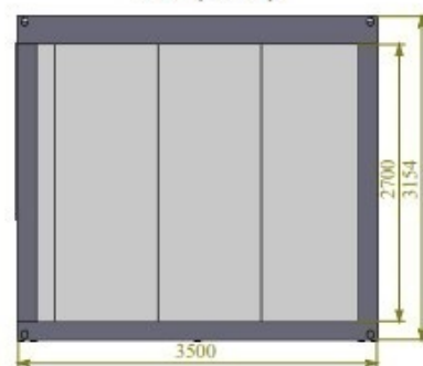
B-B (1 : 55)
