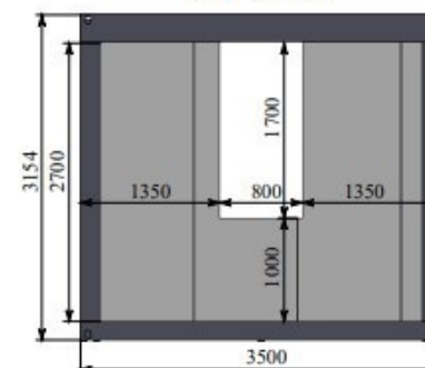
D-D (1 : 55)
