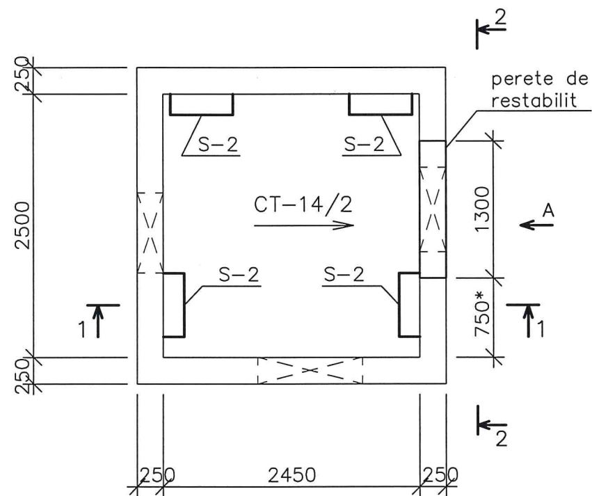
Planul caminului CT-14/1a
