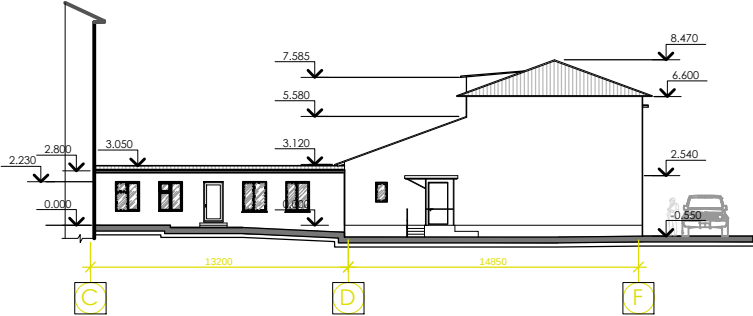
Fațada in axele C-F (existenta) sc 1:200
