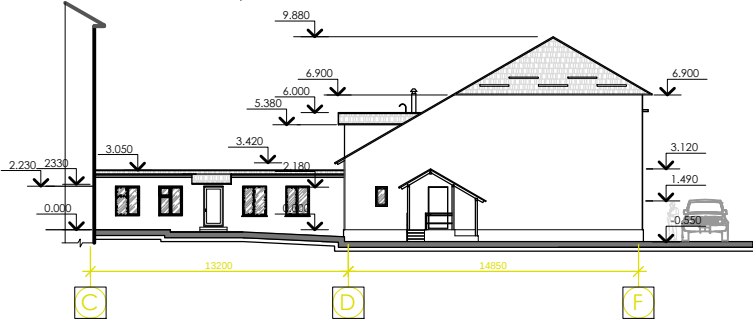
Fațada in axele C-F (propusa) sc 1:200
