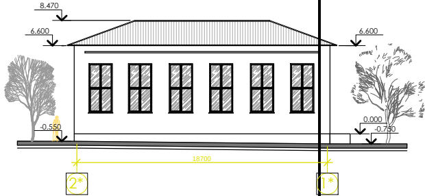
Fațada in axele 2*-1* (propusa) sc 1:200
