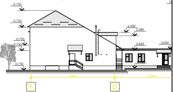
Fațada in axele F-A (propusa) sc 1:200
