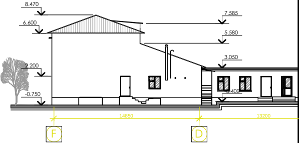
Fațada in axele F-A (propusa) sc 1:200
