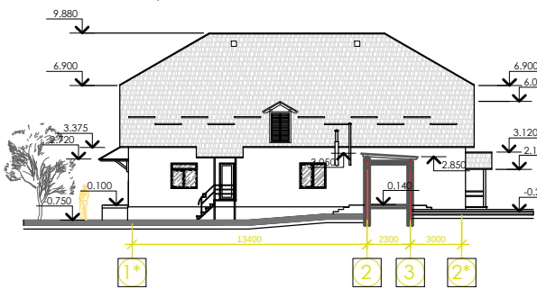
Fațada in axele 1*-2* (propusa) sc 1:200
