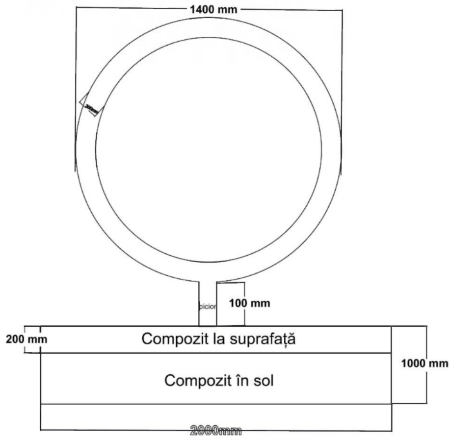
Imagine 2: Structura de susținere.
