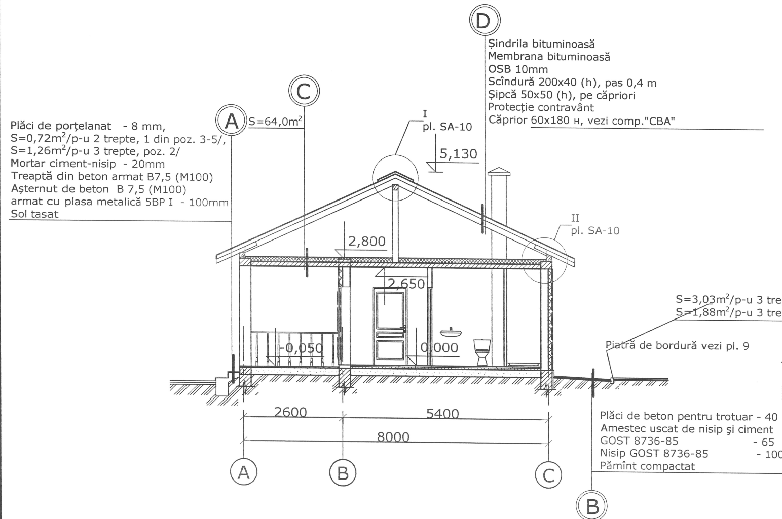
Secțiunea 1-1 /poz. 2-5/
