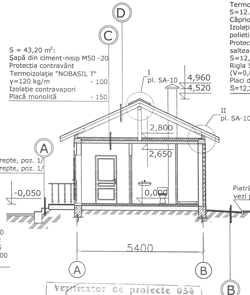
Secțiunea 2-2 /poz. 1/
