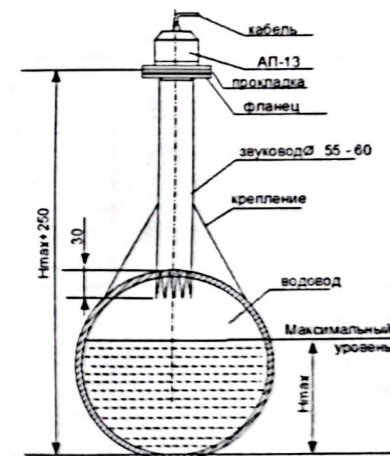
Схема монтажа расходомера ЭХО-Р-02 в комплекте с акустическим датчиком АП-13 для измерения расхода сточных вод.
