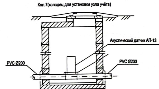
Схема монтажа расходомера ЭХО-Р-02 в комплекте с акустическим датчиком АП-13 для измерения расхода сточных вод.
