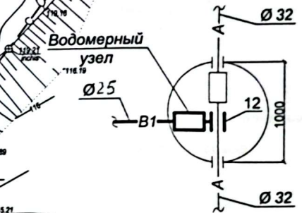
Схема установки водомерного узла Ø15 мм в колодце Кол.сущ.3
