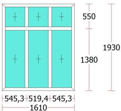
Fereastră03 - 1 buc.
