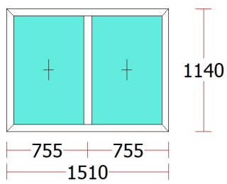
Fereastră09 - 1 buc.
