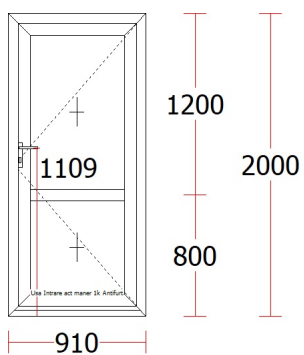
Ușă05 - 1 buc.
