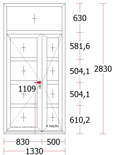
Ușă06 - 1 buc.
