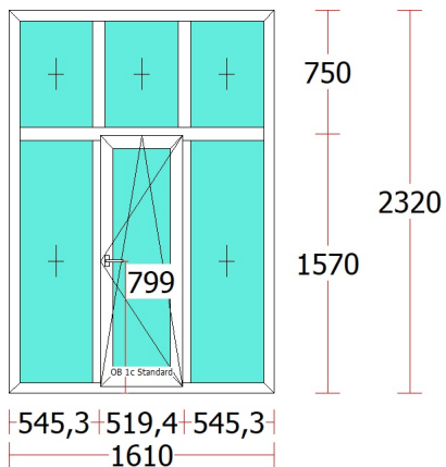
Fereastră01 - 6 buc.
