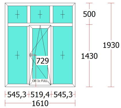
Fereastră10 - 4 buc.
