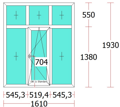
Fereastră02 - 1 buc.
