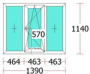
Fereastră04 - 3 buc.
