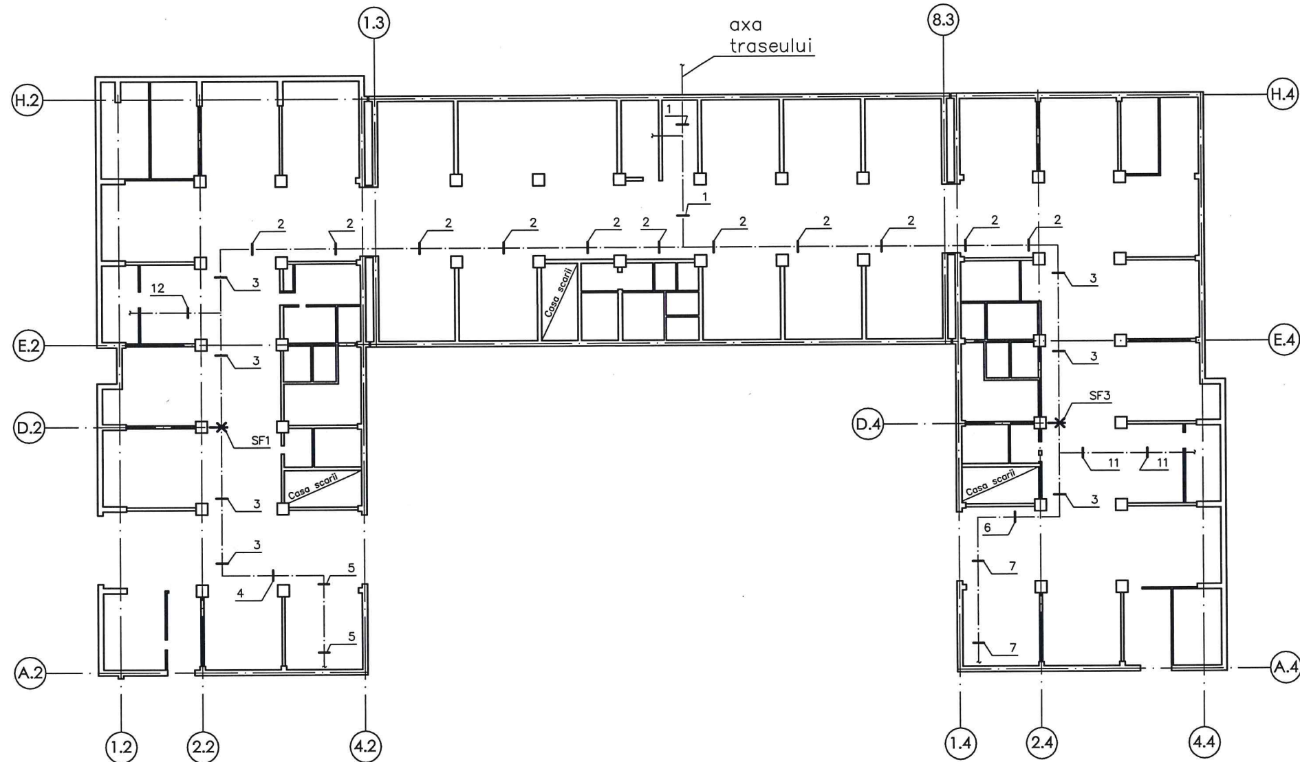
Specificatia suporturilor la nivelul -4,500
