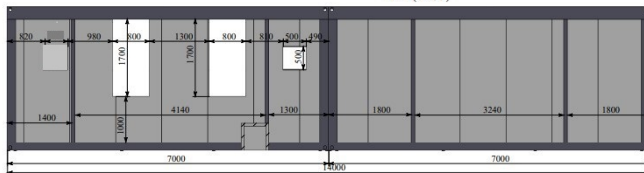
A-A (1 : 55)
