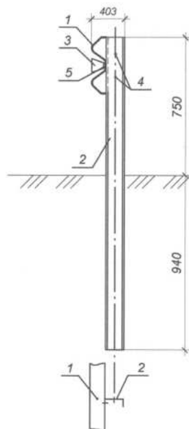
Grindă (1:20)
