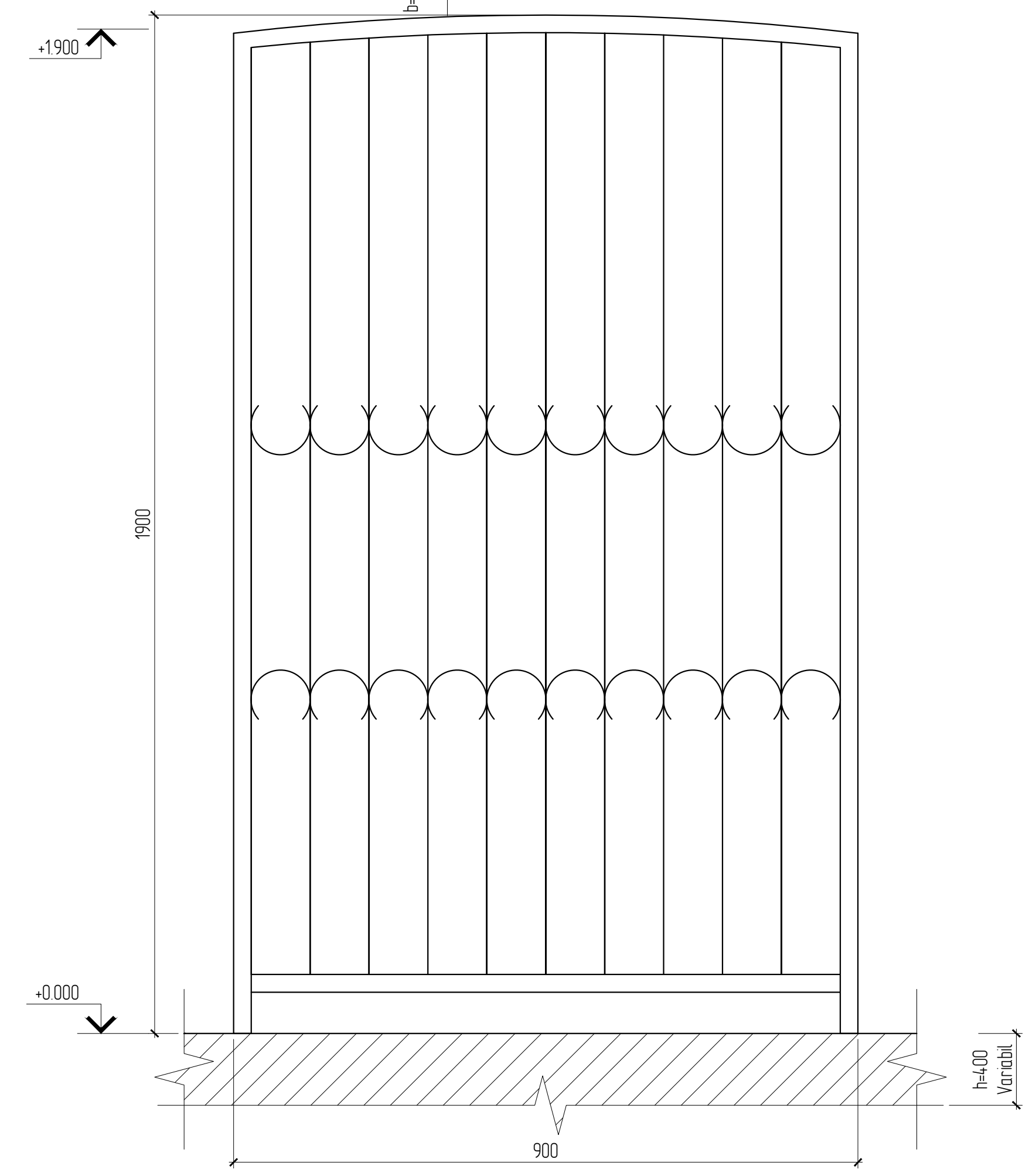
Schita-Portita Sc. 1:10
