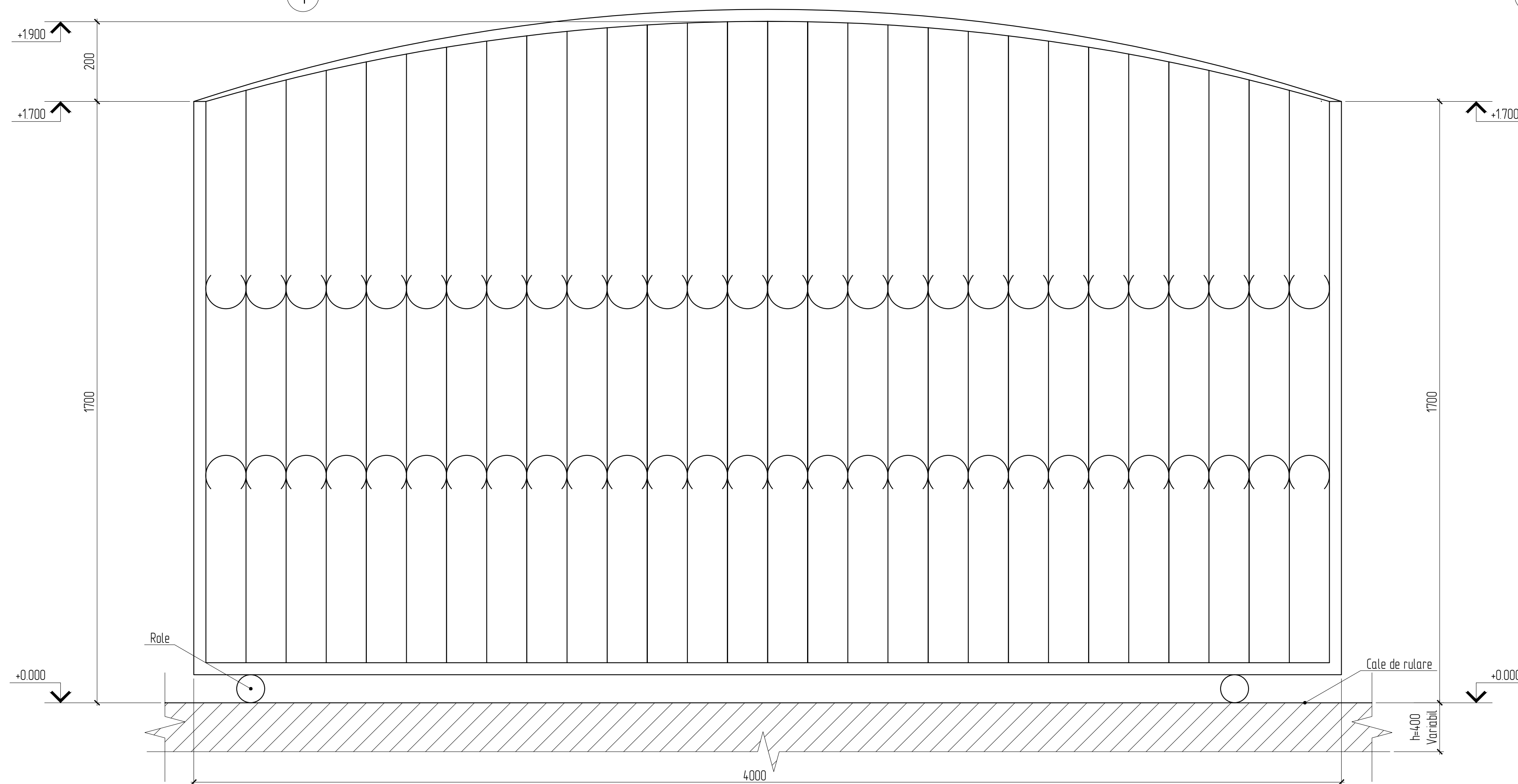
Schita-Poarta Sc. 1:10
