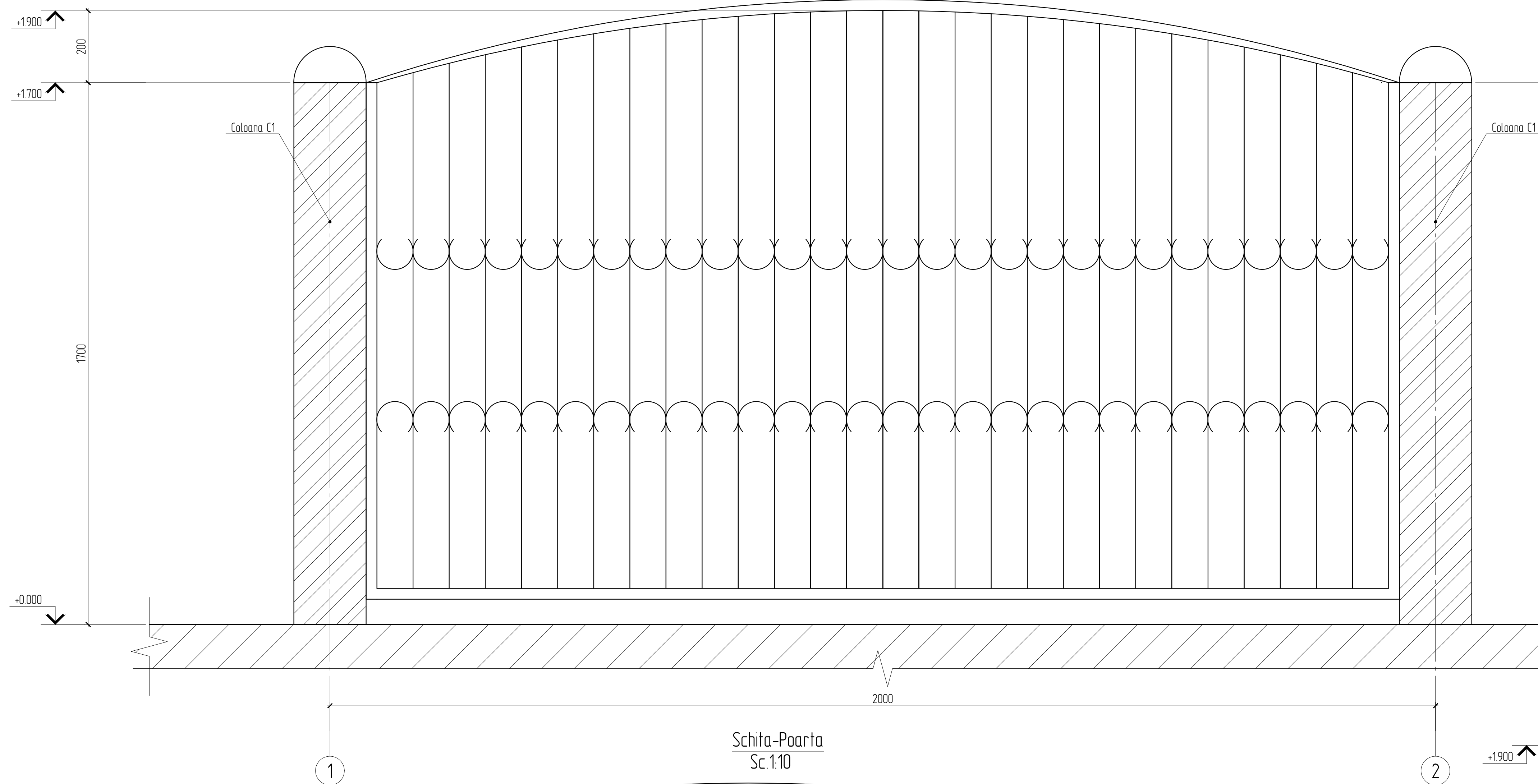
Schita-Gard Sc. 1:10
