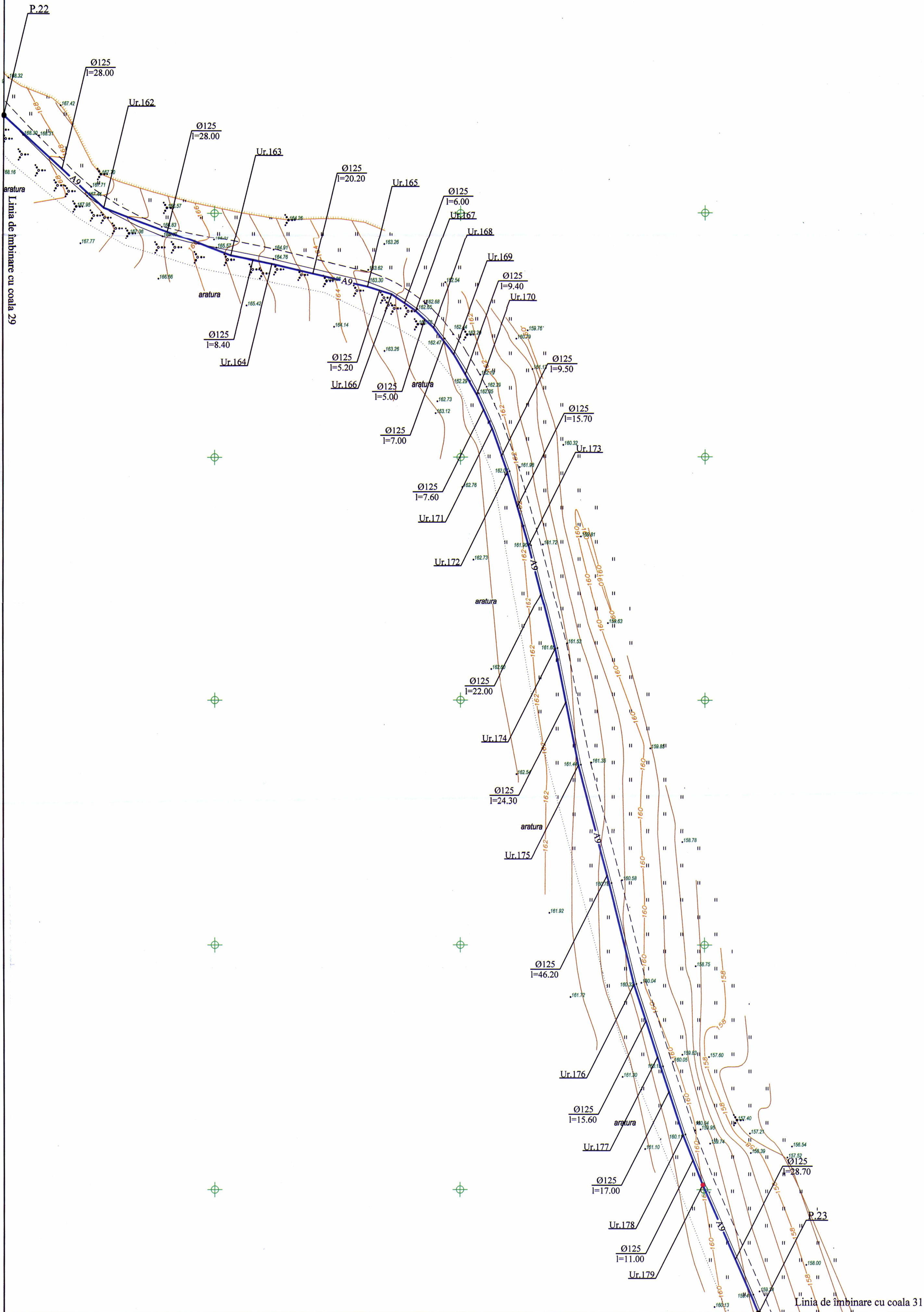
Planul rețelelor exterioare de alimentare cu apă
