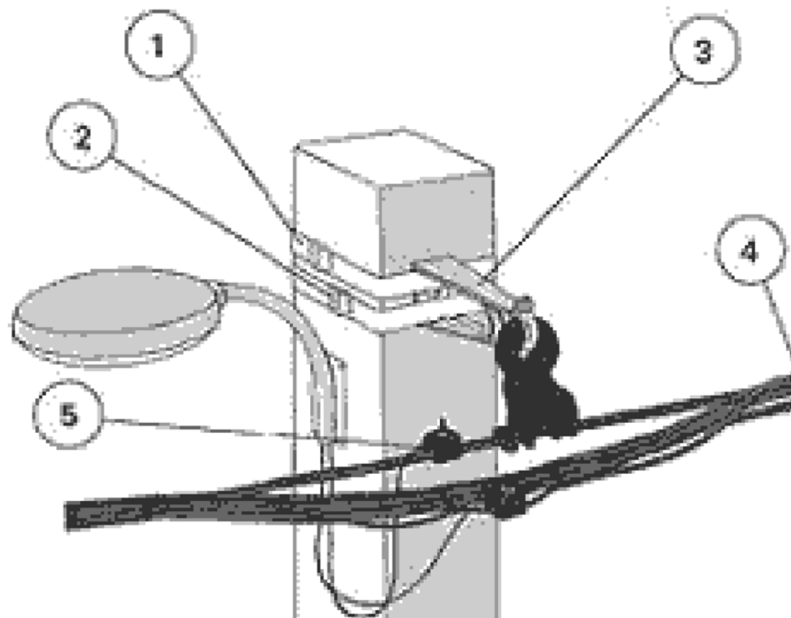
Fig.1 Armatură intermediară CИП-2 și conectarea iluminatului stradal Materiale necesare:
