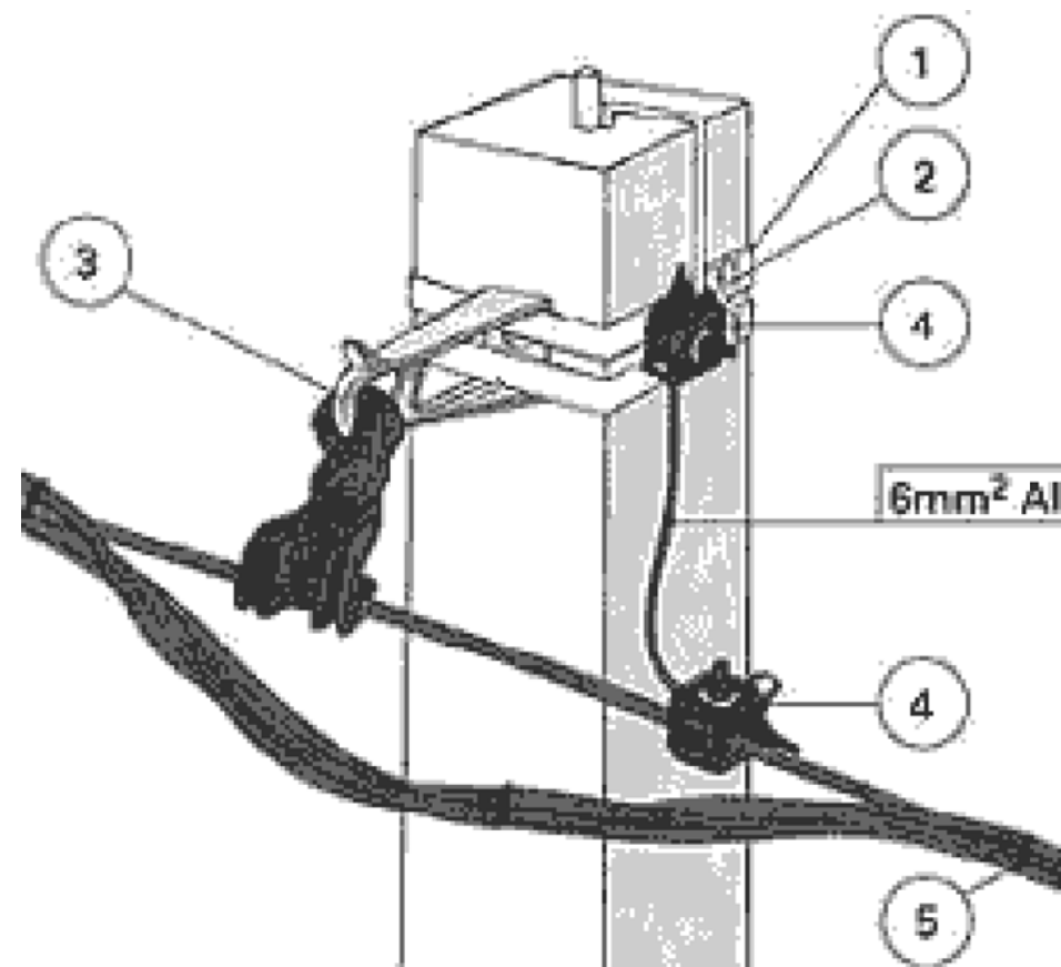
Fig.2 Armatură intermediară CИП-2 și armatură pentru legarea repetată la pământ a firului PEN
