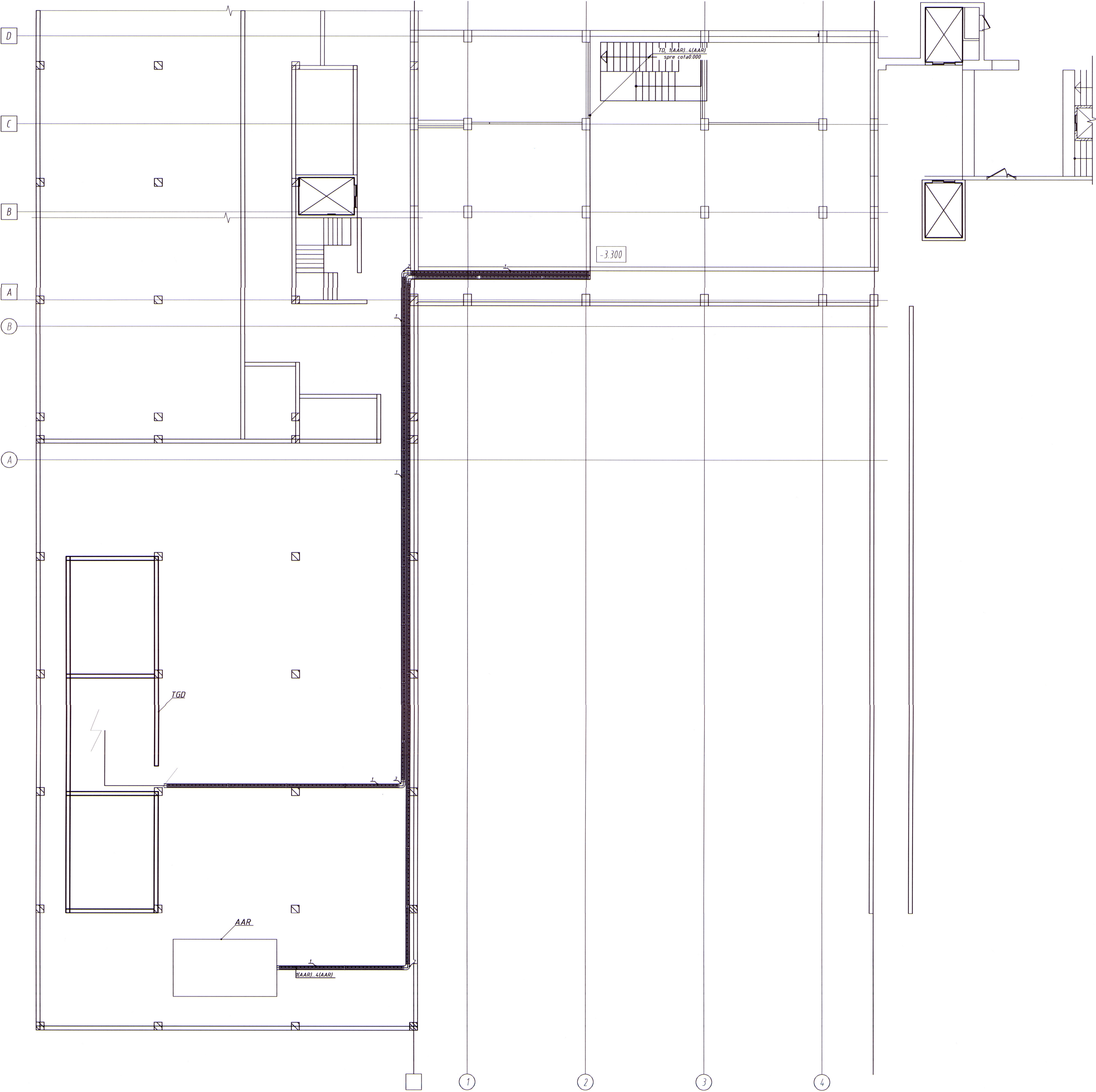
Plan Etaj la cota -3.300 Sc.1:100
