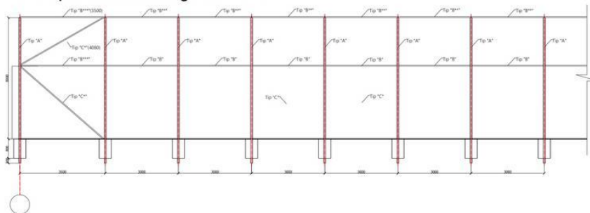
Exemplu desfasurata gard H=2m
