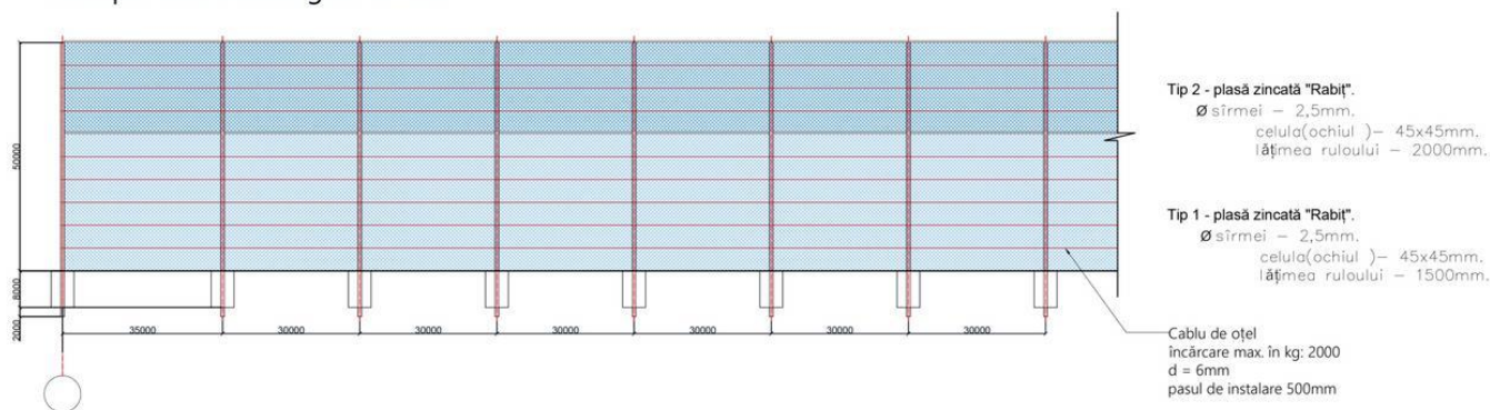
Exemplu desfasurata gard H=5m
