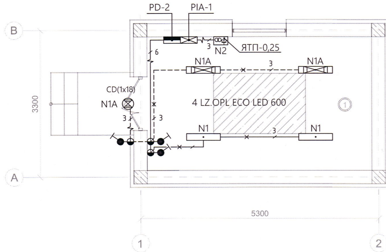
Plan echipament de iluminat la cota. 0,000. Scara 1:50
