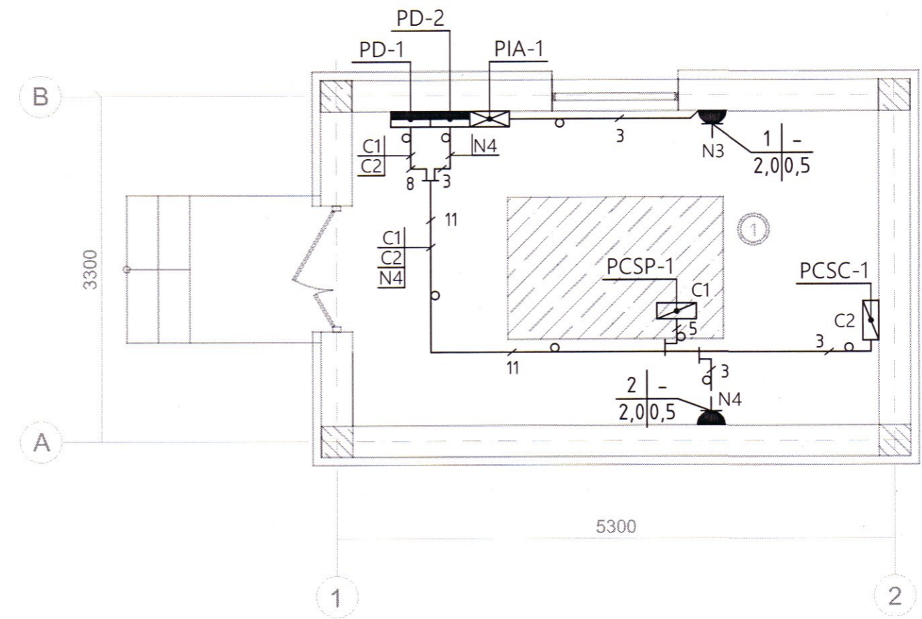
Plan echipament de forță la cota. 0,000. Scara 1:50
