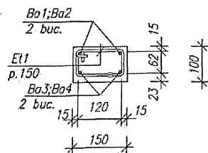
Secțiune a-a(sc.1:10) (desen de armare)
