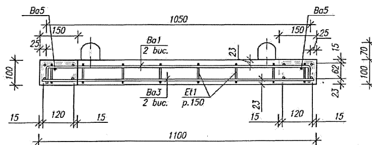
Secțiune 1-1 sc.1:10 (desen de armare)
