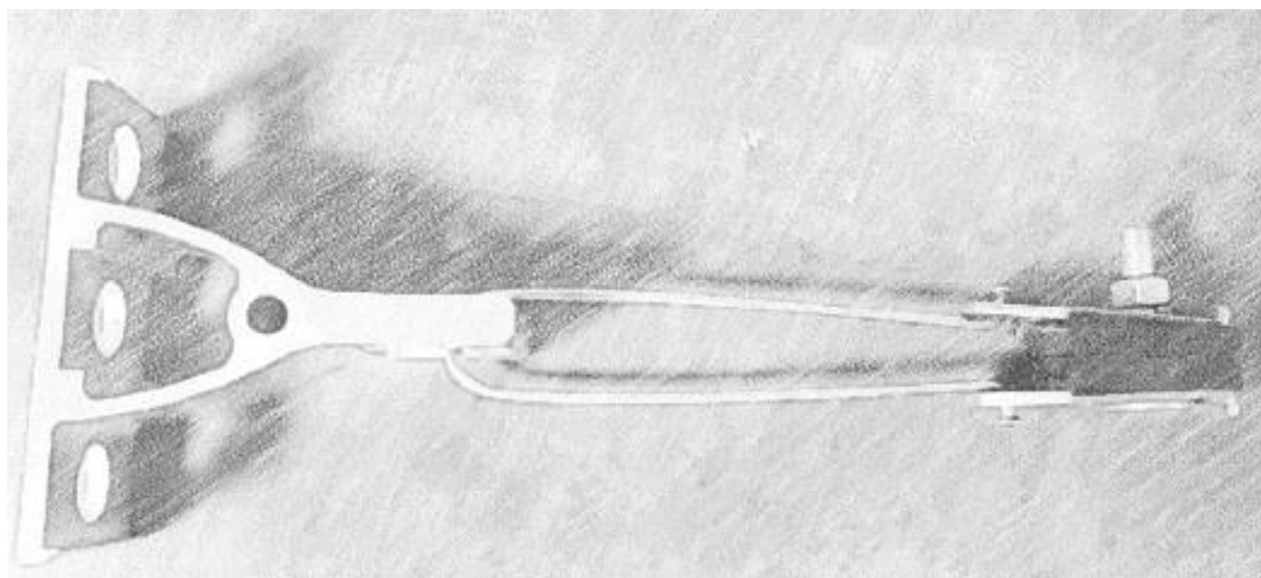
Fig.1.1 Clemă de întindere 2x35 (clemă de ancorare+suport compoziție aluminiu analogic CA1500) Figura sus prezentată are caracter informativ.
