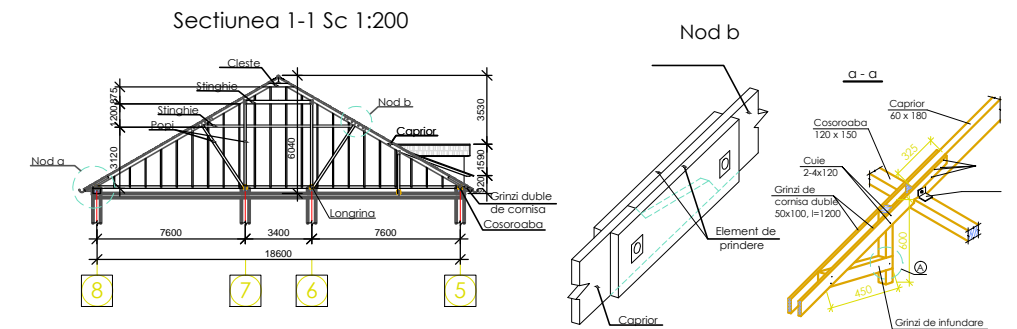
Elemente de jonctiune ale sarpantei
