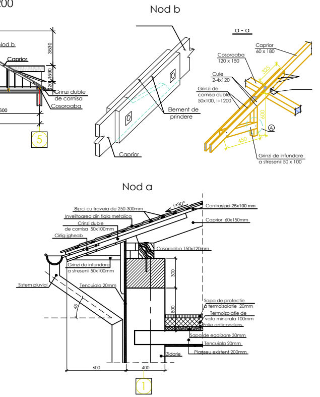
Elemente de jonctiune ale sarpantei
