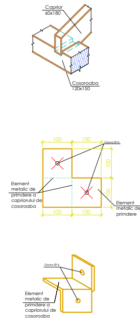
Elemente de jonctiune ale sarpantei
