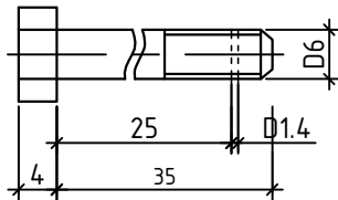
Detaliu poz.5
