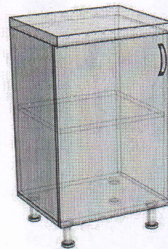
2) Tumbă cu top din blat 480x420x840(1buc.)
