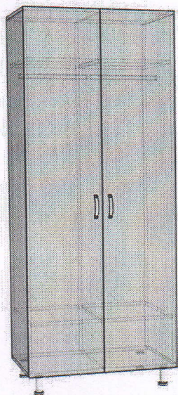
1) Dulap pentru haine 800x550x2000(2buc.)
