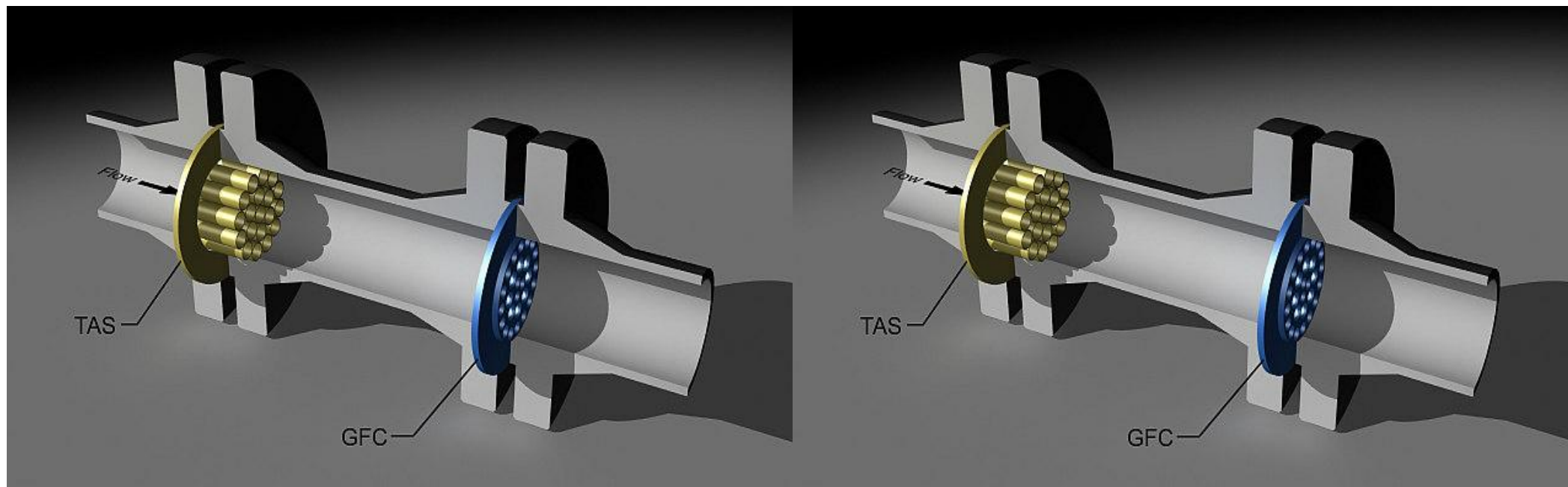
Figura 1c - Imaginea 3D a DUC Gallagher cu un dispozitiv tubular anti-vortex, unde:
