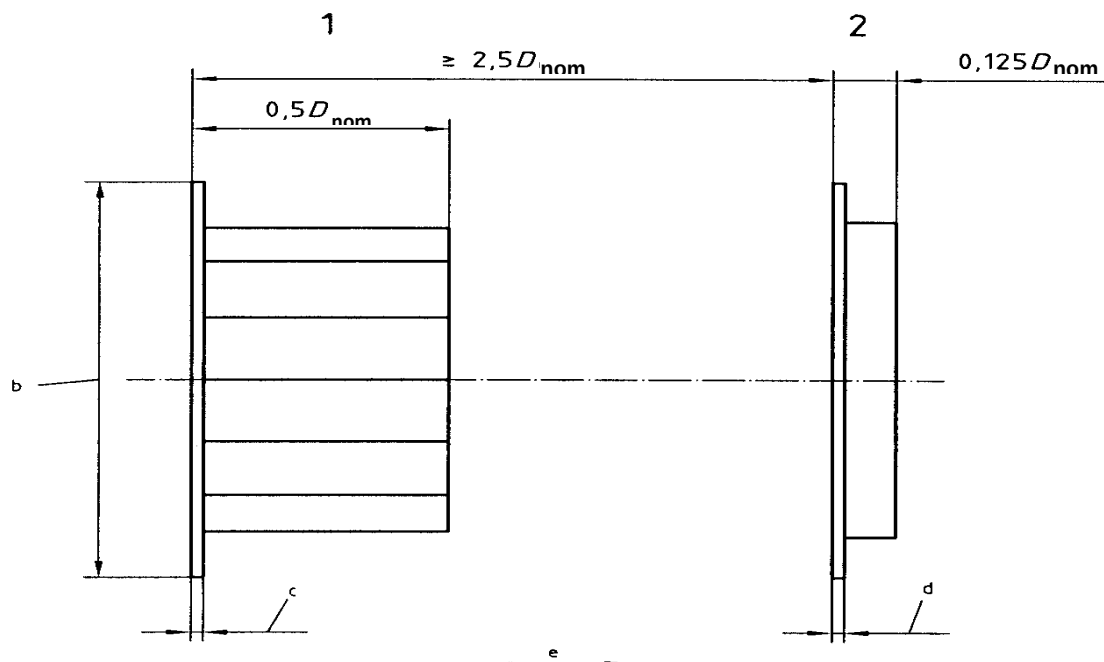
Figura 1a - Construcția caracteristică Liniștitor de flux DN500 DUC Gallagher, unde:
