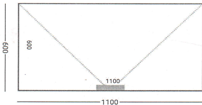
Construcție din PVC cu sticla – 1 buc.
