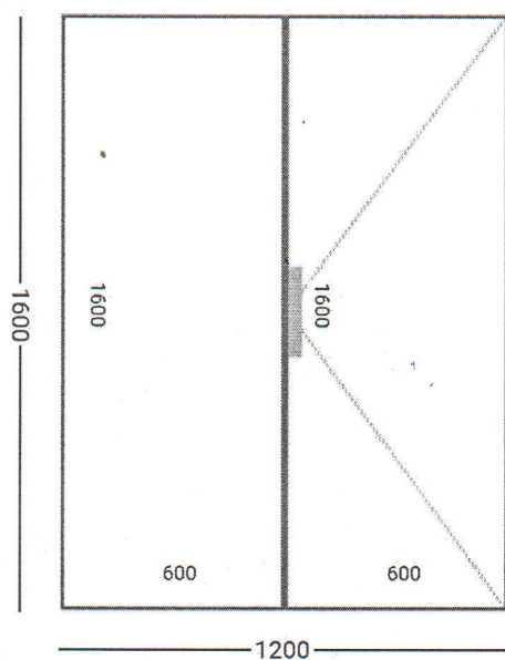
Construcție din PVC cu sticla – 6 buc.
