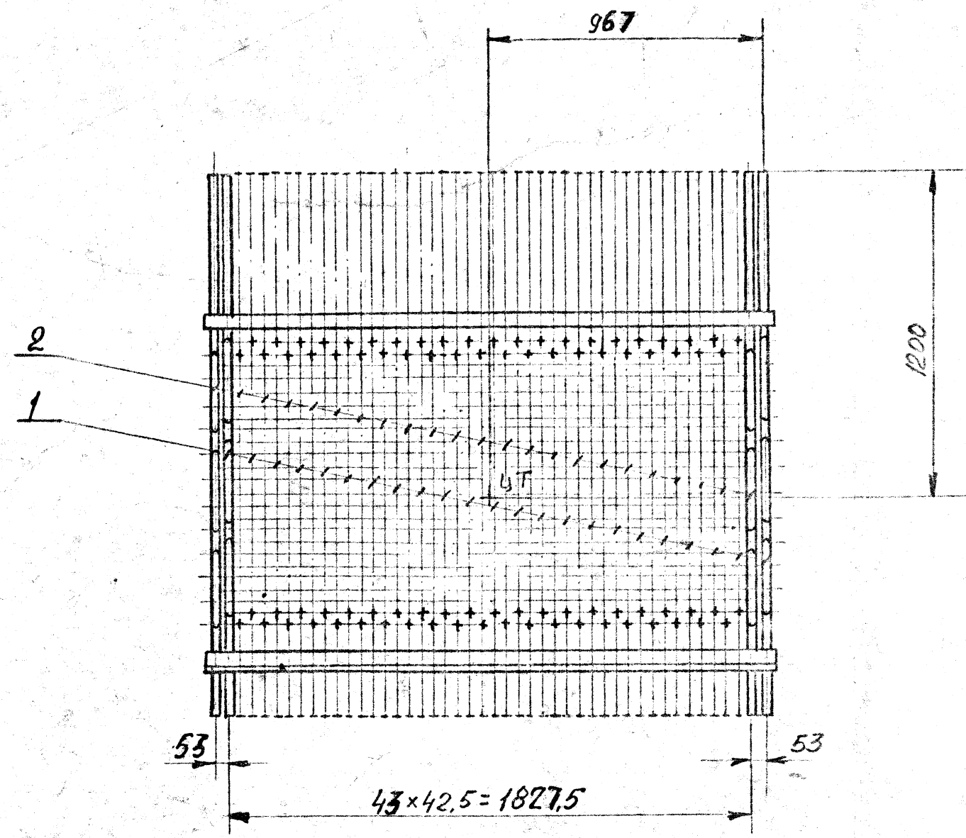
I M1:5
