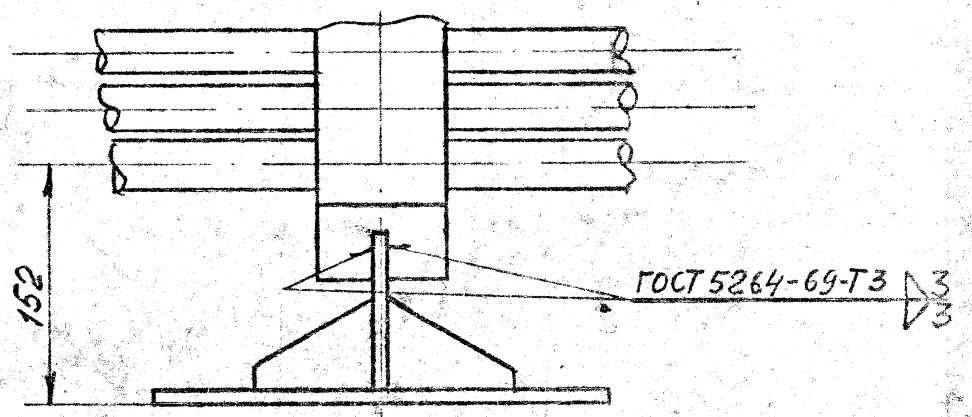
I M1:5
