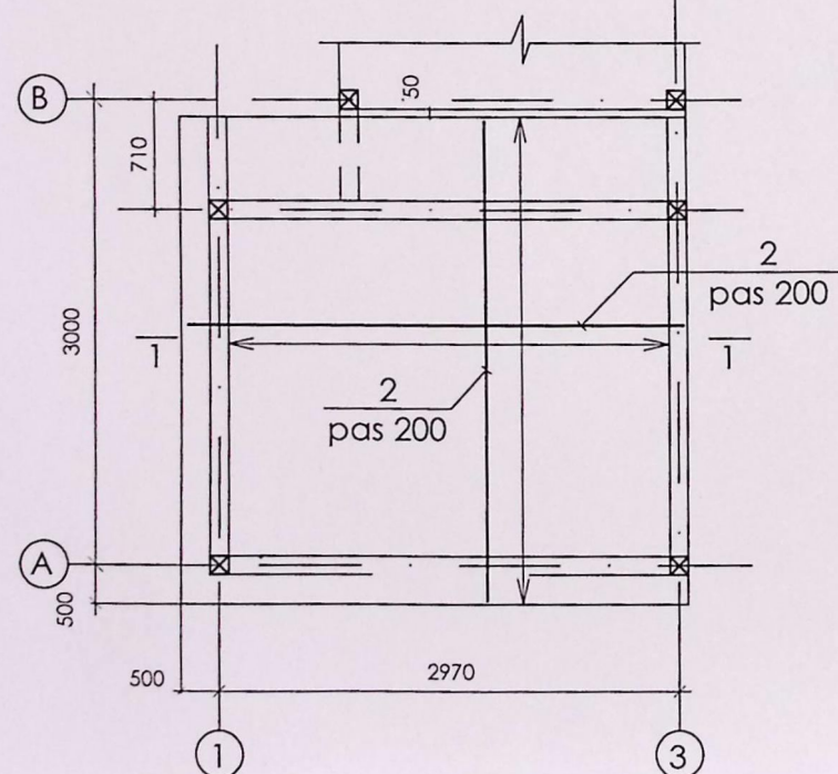
Plan planseu monolit Pm-1 niv. 2.800m (plasa de sus). sc. 1:50
