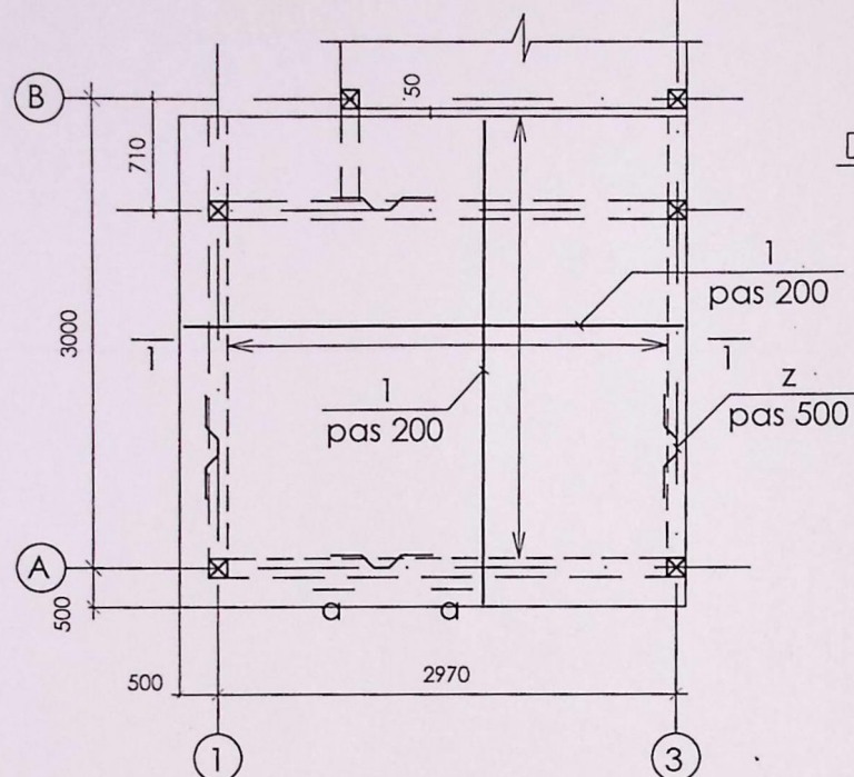
Plan planseu monolit Pm-1 niv. 2.800m (plasa de jos). sc. 1:50
