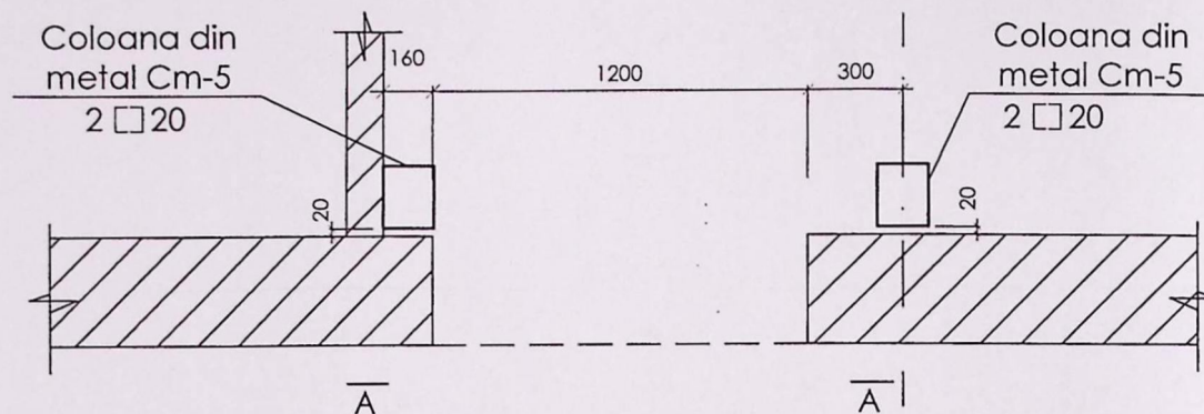
Plan de situatie a golului de usa consolidat. sc 1:20
