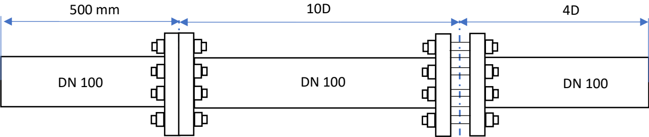
Figura 1: Segmentul conductei de măsurare DN 100 care include camera inelară și secțiuni calibrate 10D până la elementul primar (diafragmă) și 4D după.
