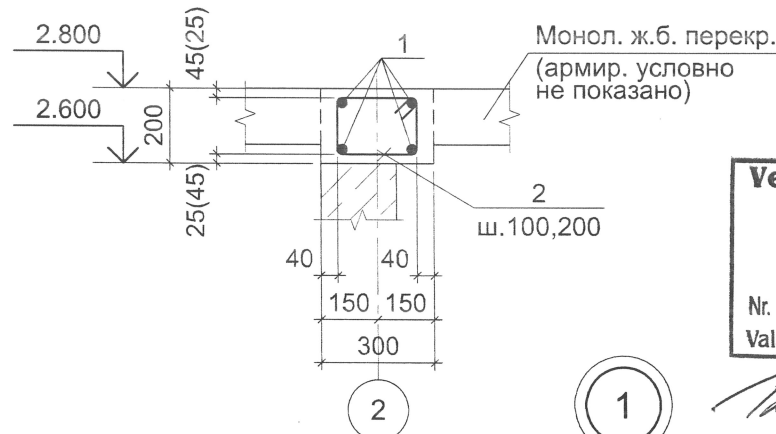
2 - 2 (Пояс ПСм-1)
