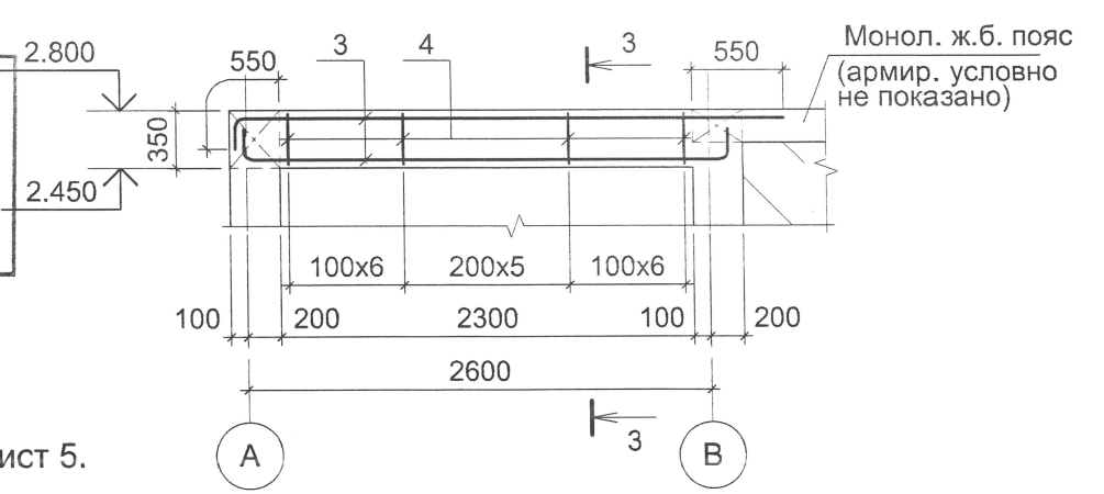
РГм-2
