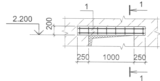
Перемычка ПРМ-1
