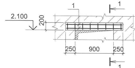
Перемычка ПРМ-2
