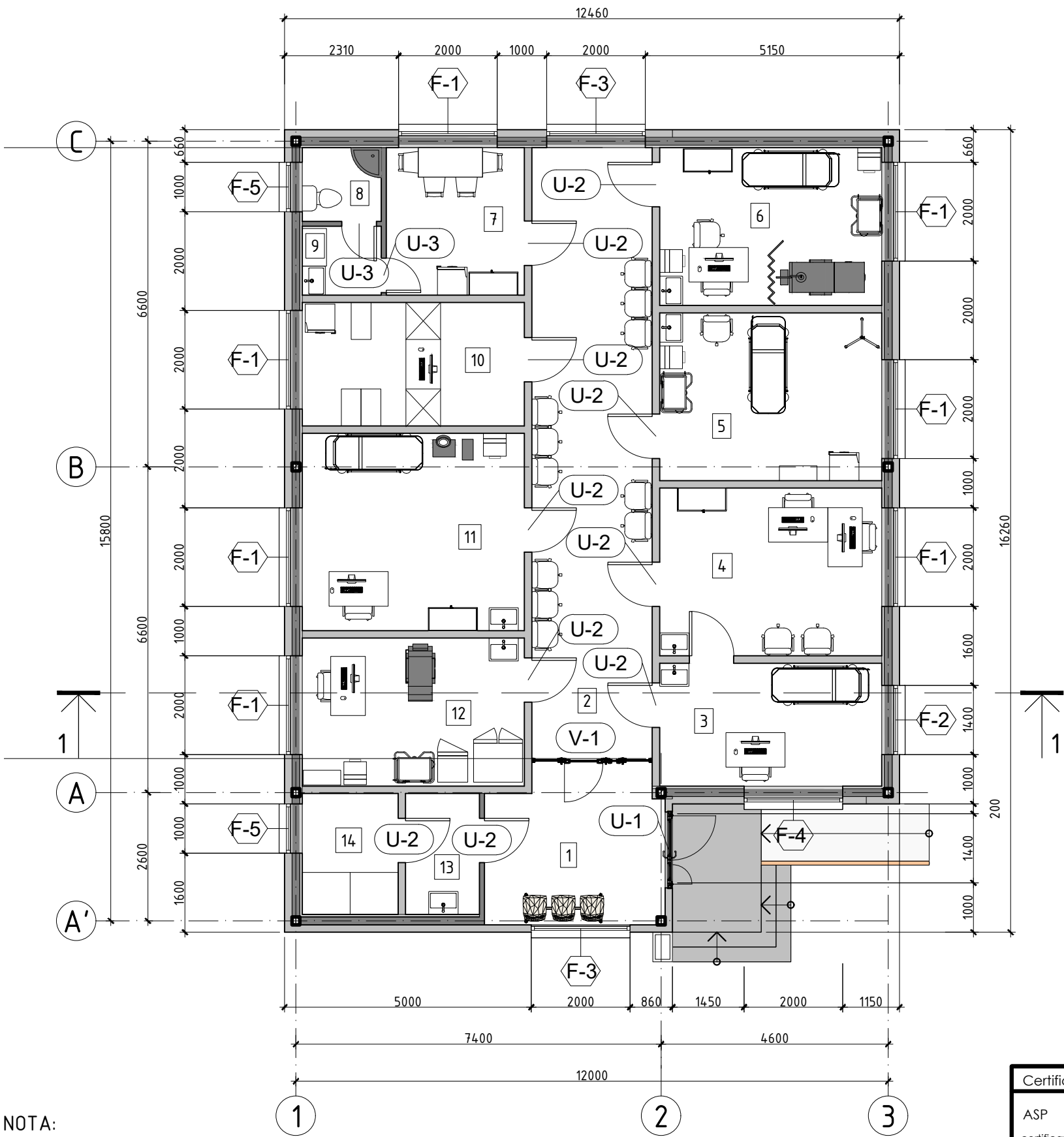
PLAN PARTER COTA 0.000,(finisari) sc.1:100
